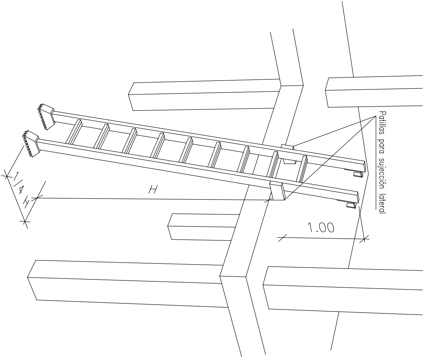
POSICION CORRECTA DE ESCALERAS DE MANO
