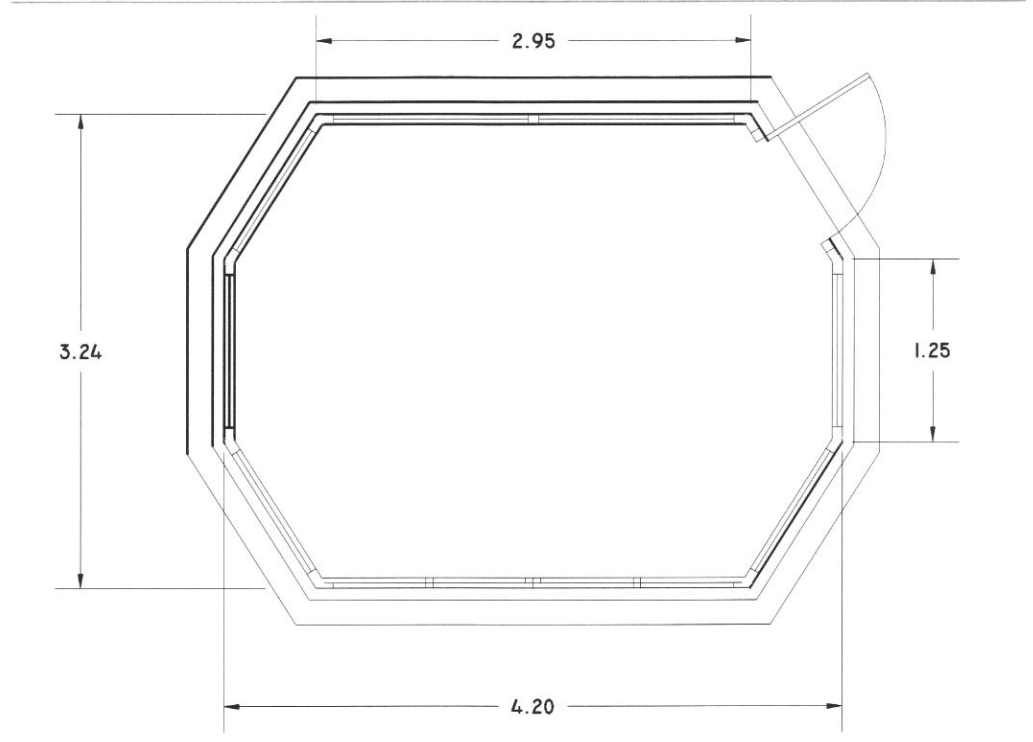
planta acotada. e_1.100
