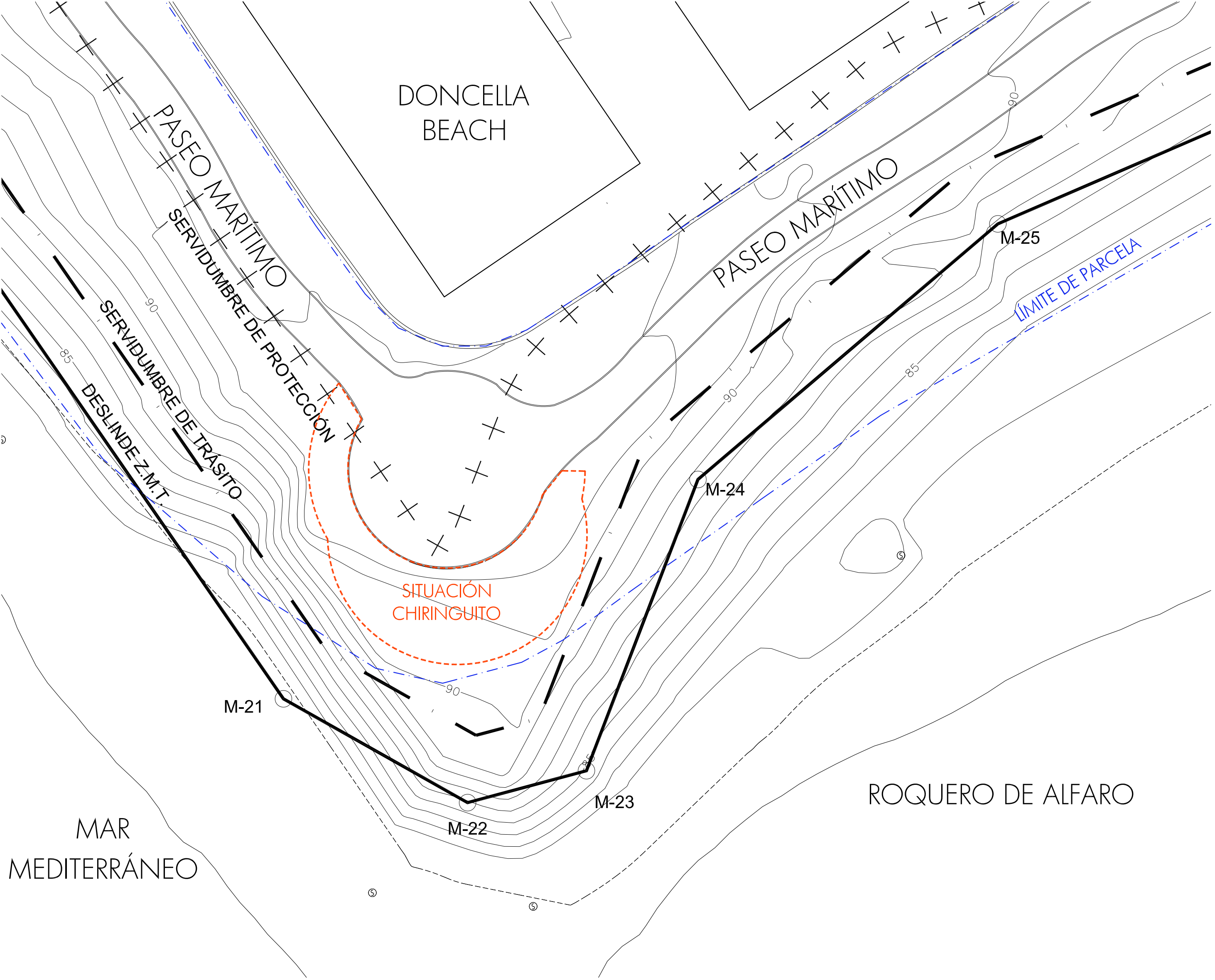
EMPLAZAMIENTO, TOPOGRAFÍA ACTUAL (1/300).
