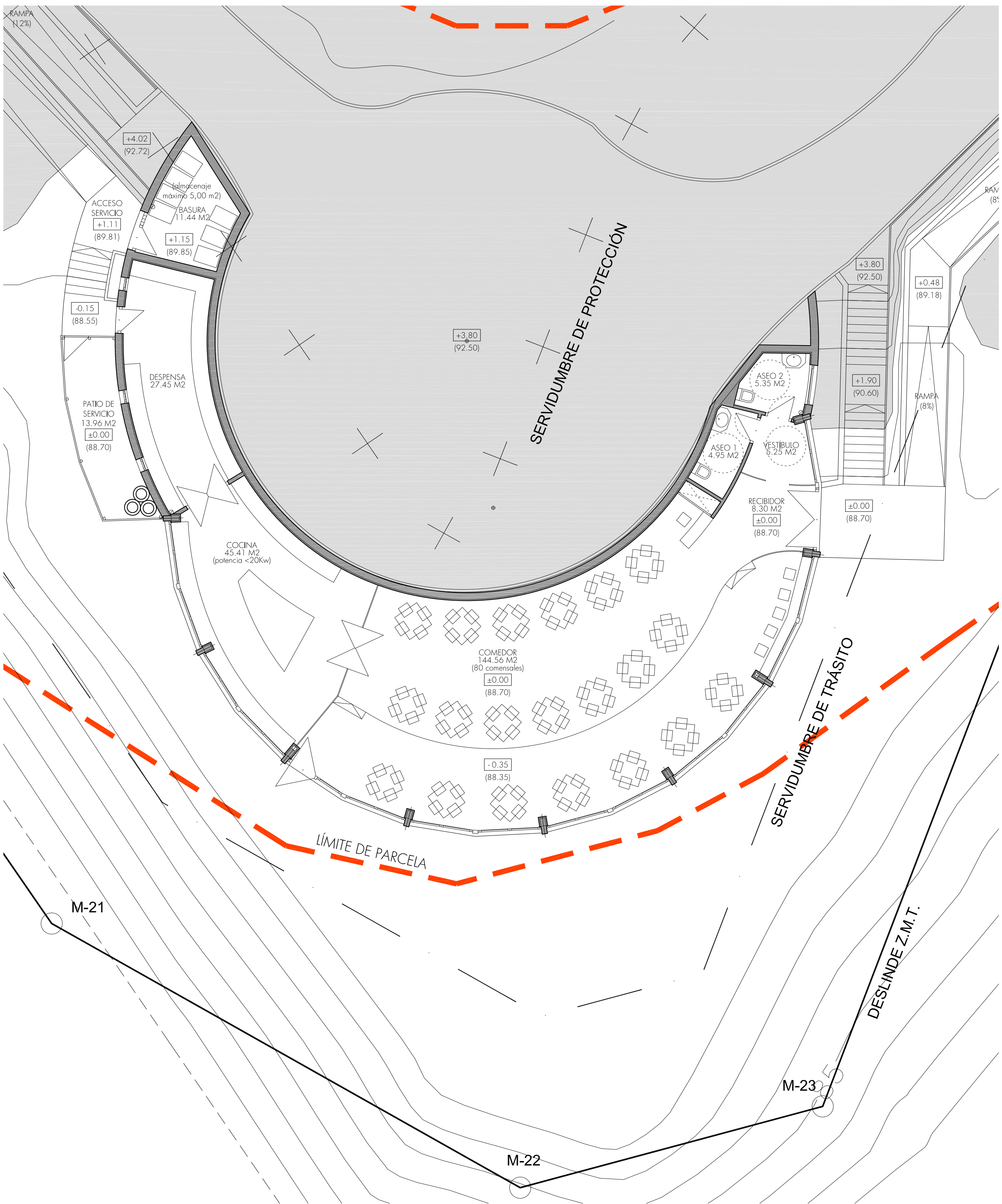
PLANTA BAJA (COTA ±0.00)
