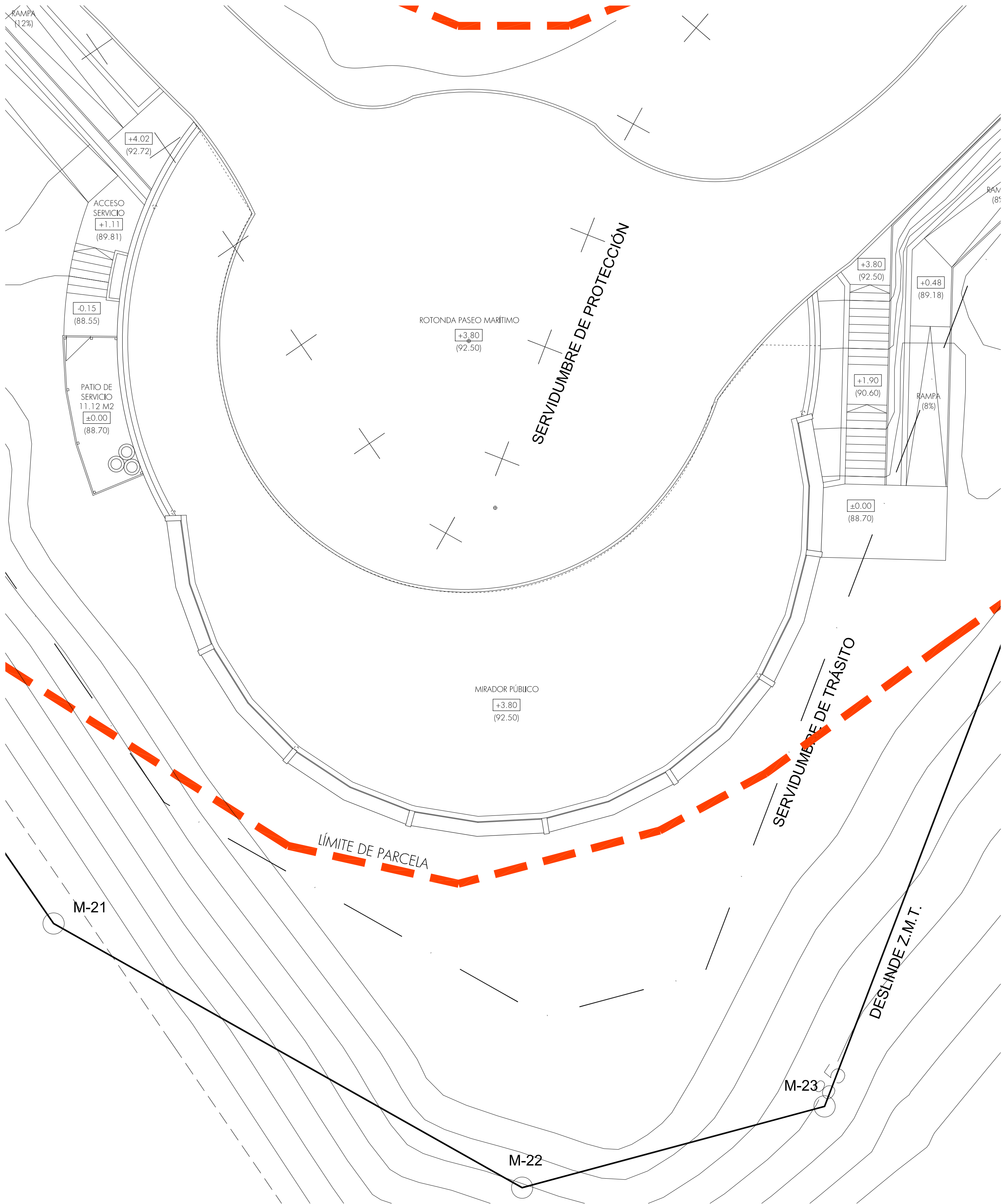
PLANTA DE CUBIERTA (COTA +3.80)
