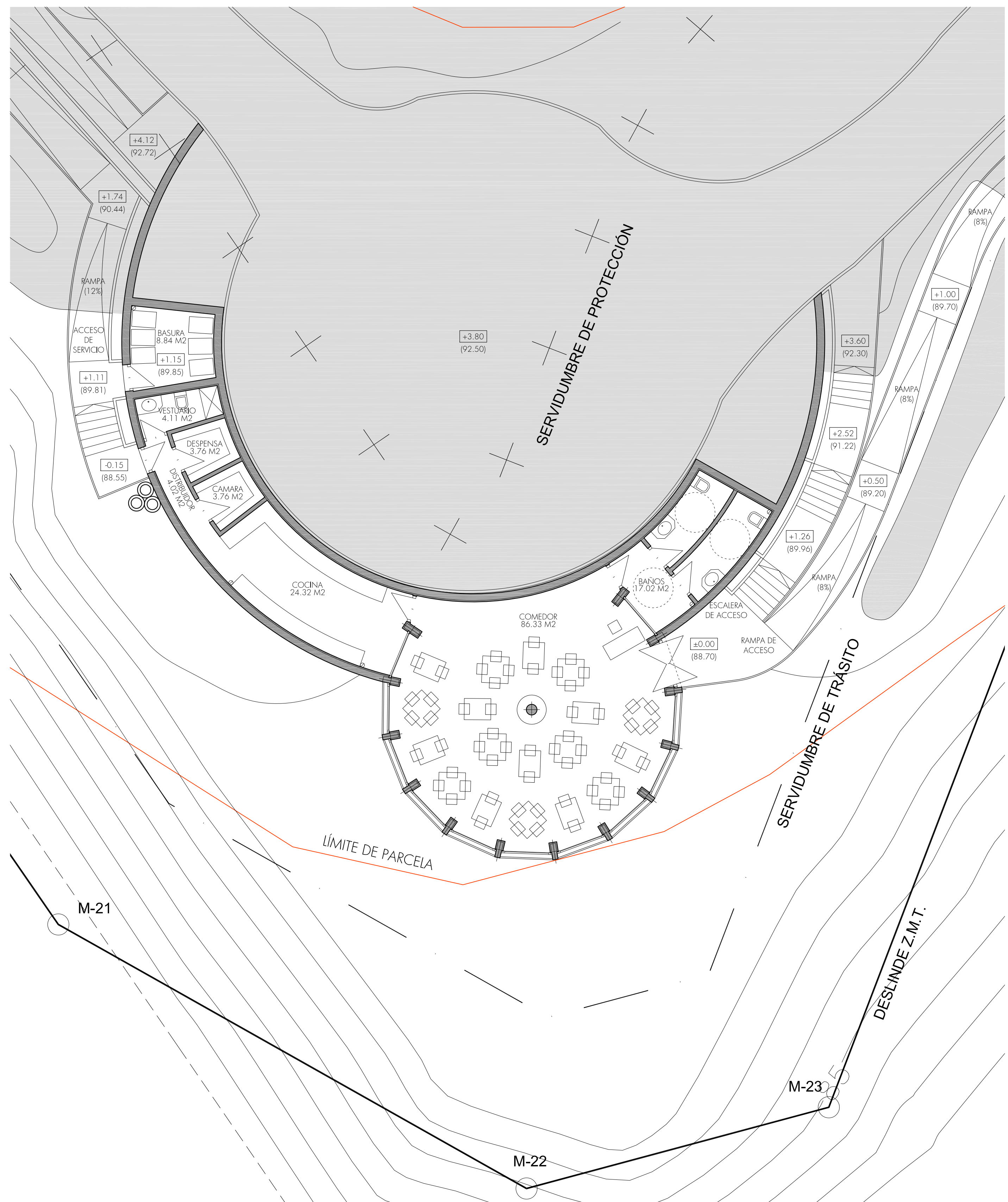
PLANTA BAJA (COTA ±0.00)
