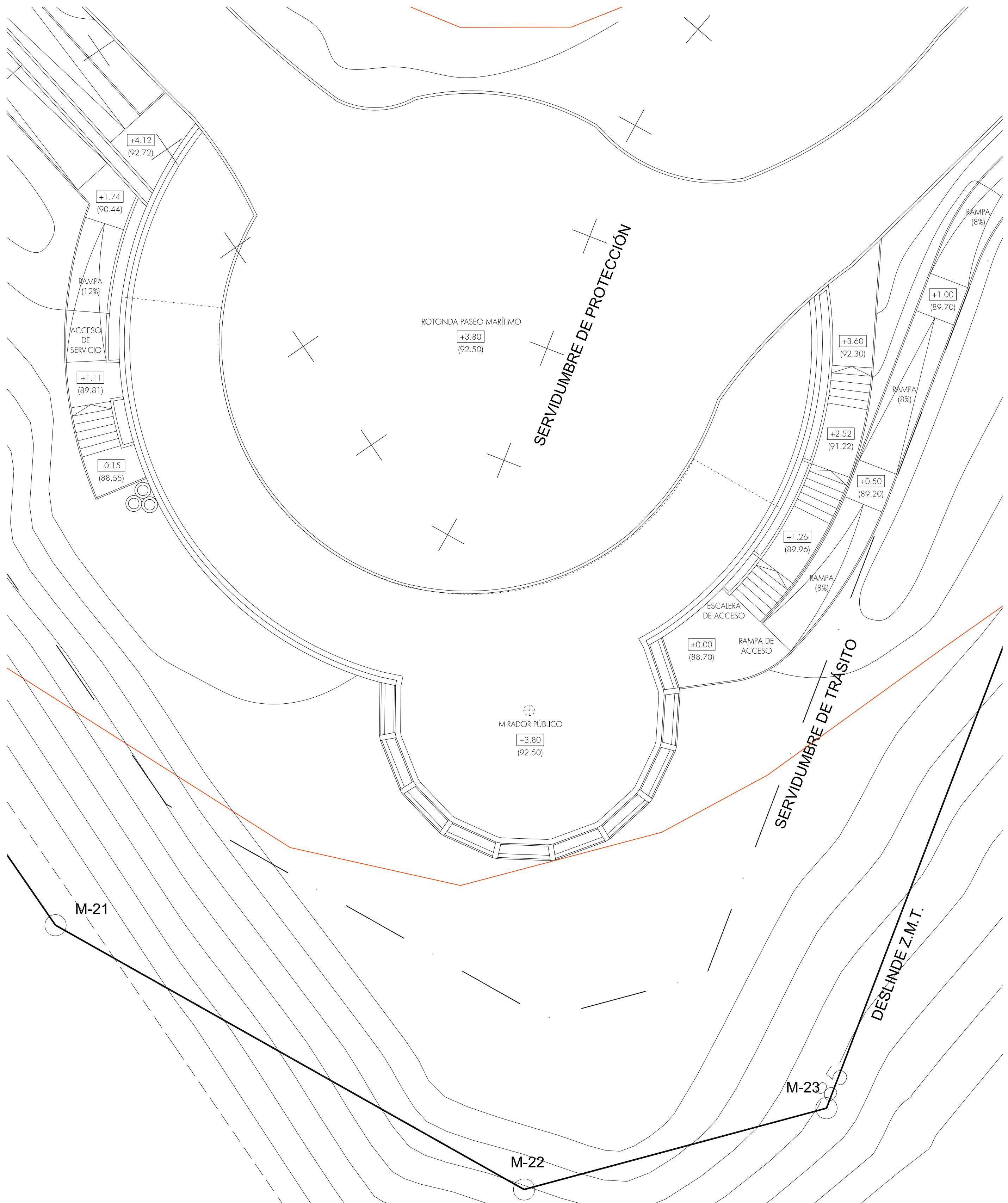
PLANTA DE CUBIERTA (COTA +3.80)
