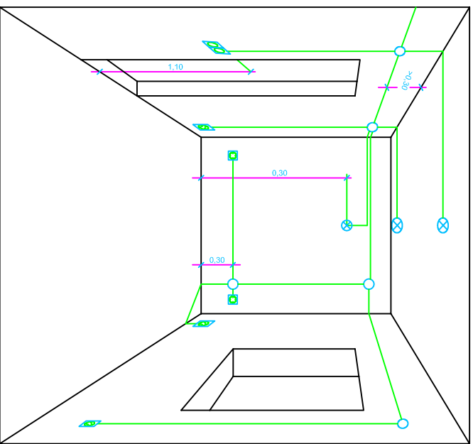
ESQUEMA DE TRAZADO DE CANALIZACIONES
