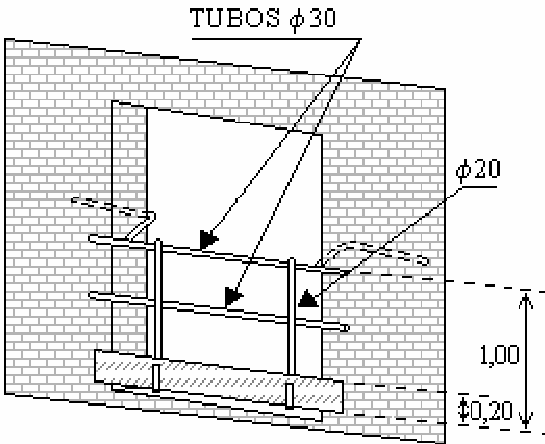
BARANDILLA DE HUECOS VERTICALES
