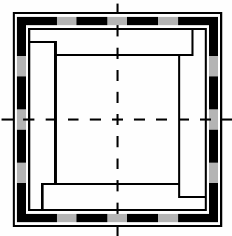
ENTIBACIÓN EN CUADRO DE MINA
