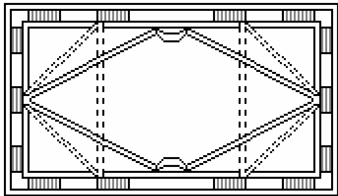
ENTIBACIÓN DE POZOS RECTANGULARES CON MARCO DE JABALCONES
