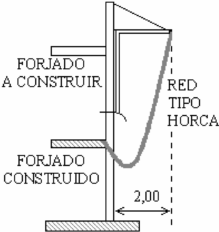
ESQUEMA DE DISPOSICIÓN DE RED VERTICAL
