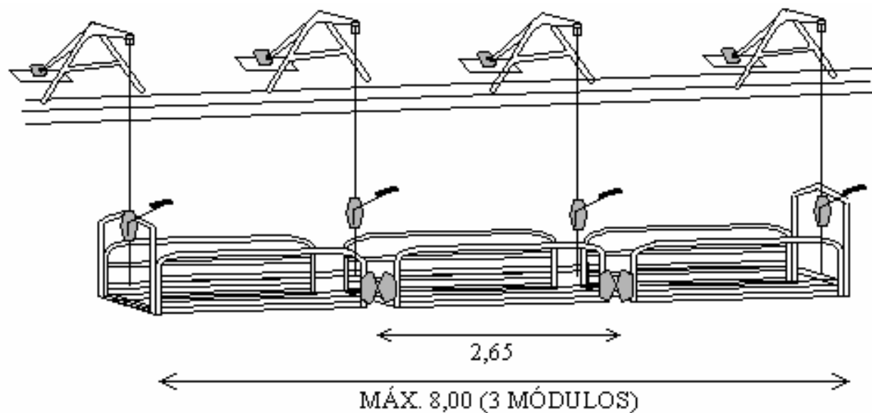
DISPOSICIÓN GENERAL DE ANDAMIOS COLGADOS
