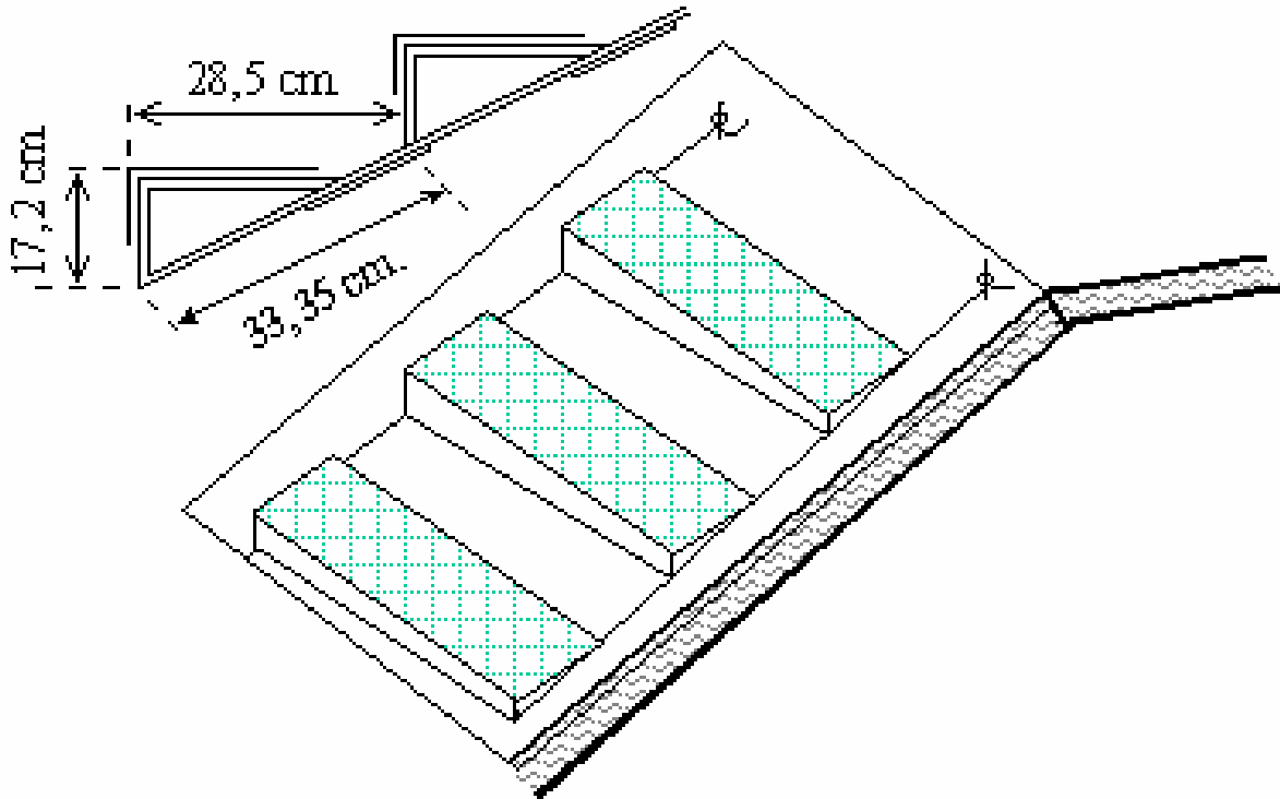
ESCALONES CON ENGANCHE
