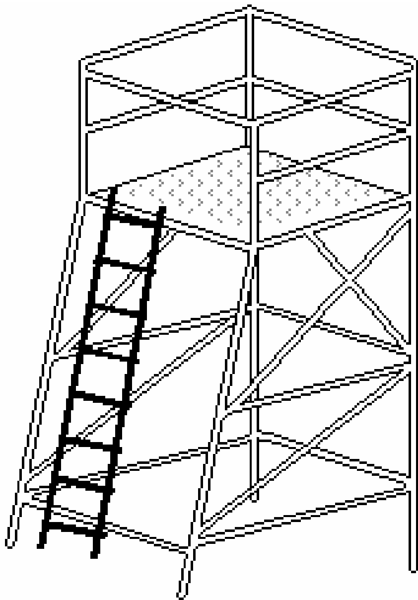
CASTILLETE METÁLICO
