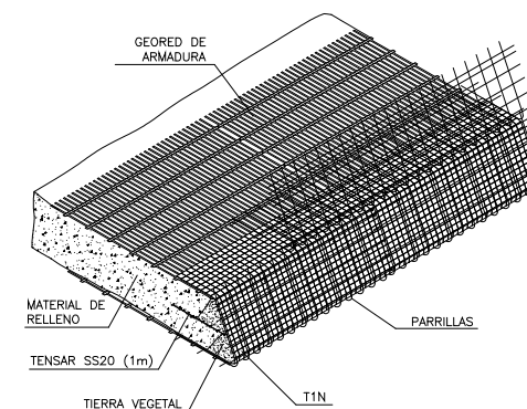
DETALLE MURO VERDE TECONMA
