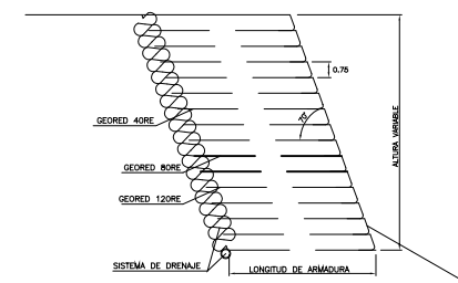
SECCION TIPO MURO VERDE ESCALA 1/200
