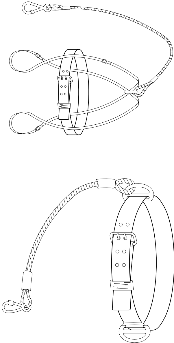
CINTURON DE CAIDA
