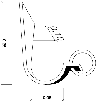
GANCHO
