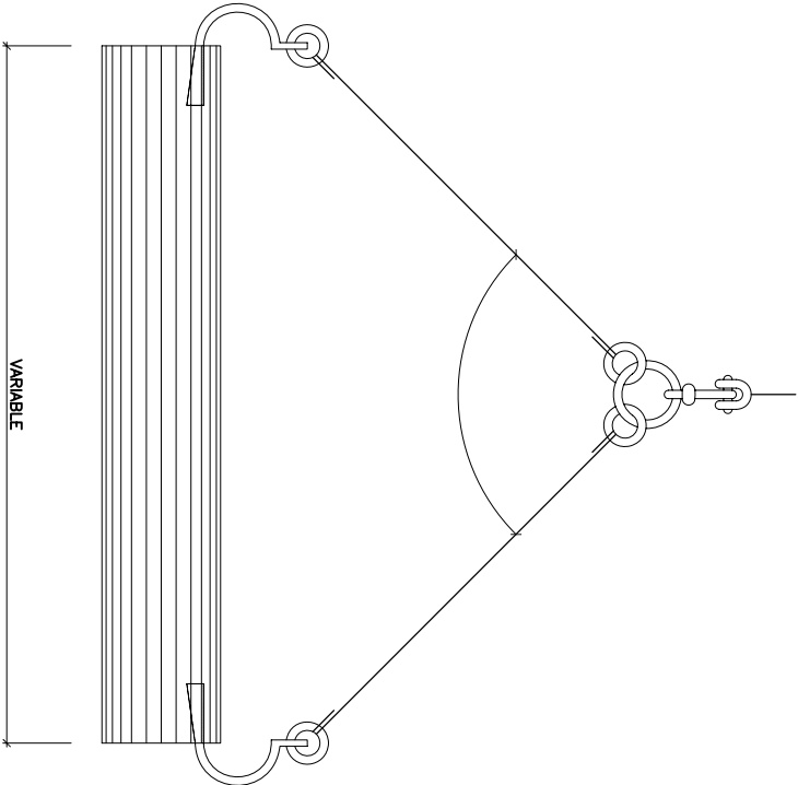
TRASLADOS DE TUBOS
